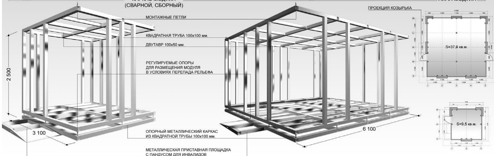
ПЛАН МОДУЛЯ
