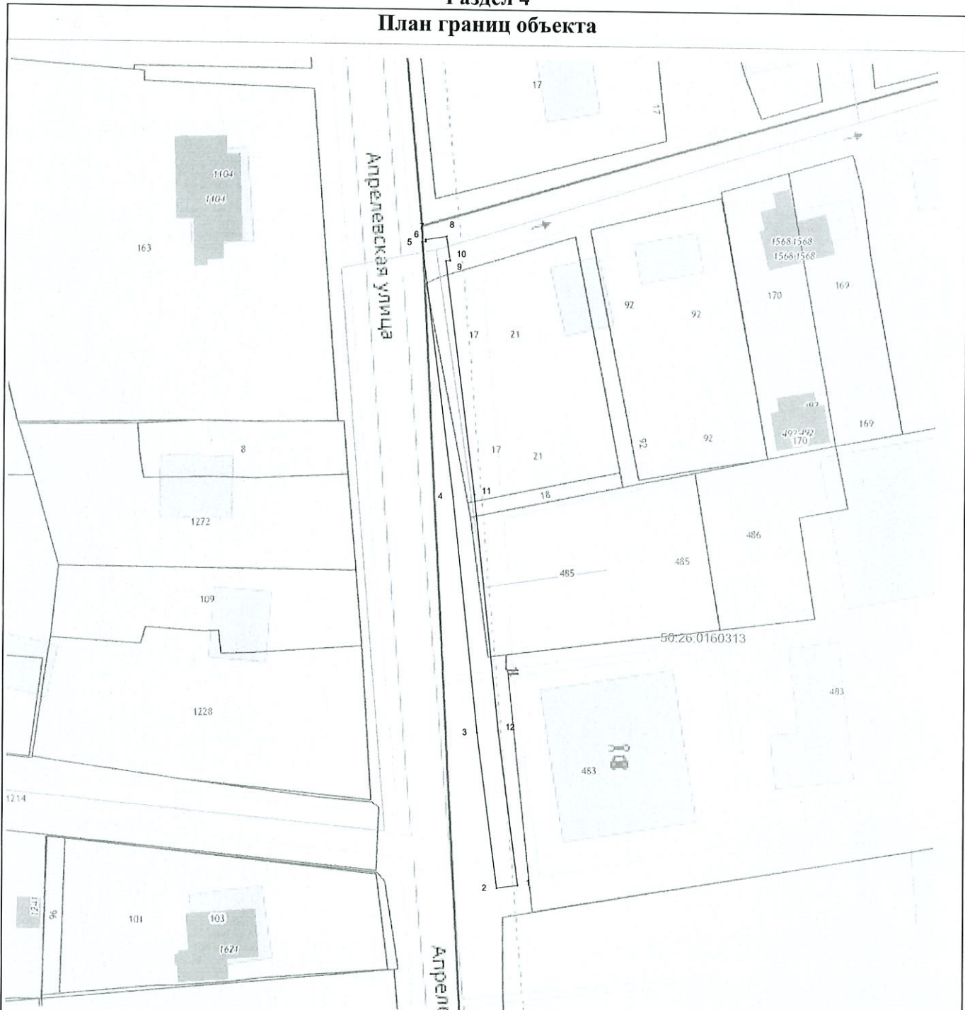
Масштаб 1:1 000
